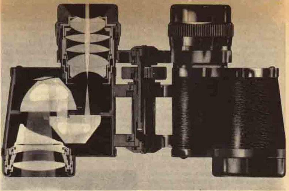
Prizmalı bir dürbünün yarısının, kesit olarak gösterilmesi.
