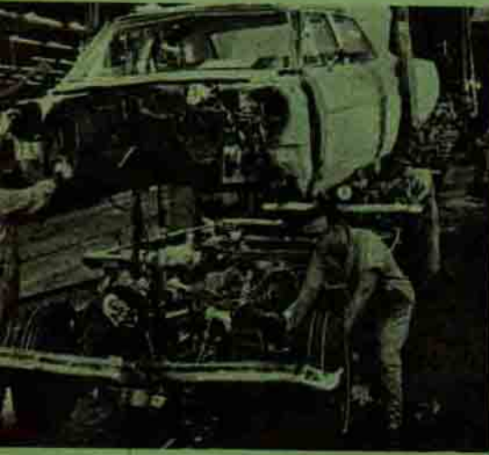
Karoserinin şasiye oturtulması en fazla heyecan veren anlardan biridir.
