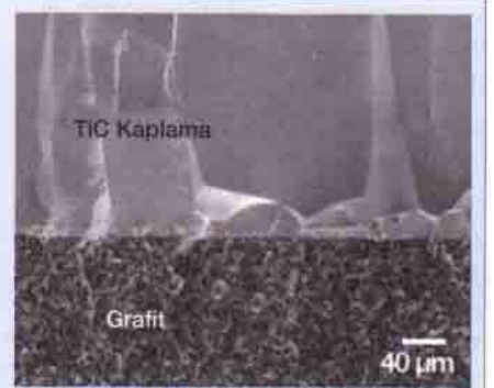
Üstte POCO AXF = 50 grafitinin 150 mikrometrek titanyum karbid (TiC) kaplaması görülüyor. Bu kaplamanın kalınlığı birkaç mikrometreden, 250 mikrometreye kadar ayarlanabiliyor.
