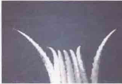
Titanyum tetraklorid (TiCl 4 ) gösteri uçuşu yapan uçaklarda havada iz bırakmak için kullanılıyor
