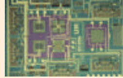
Basınç ve sıcaklık ölçümü için yapılmış bir MEMS. Mor bölgelerde mekanik diyaframlar ve sıcaklık sensörleri, geri kalan bölümdenyse tümüyle elektronik devreler vardır.
