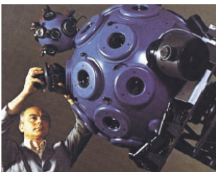
Planetaryumların mutfağı. Modern planetaryumlardaki projektörler çoğunlukla hidrolik bir asansörle salondan alt kat-taki bakım salonuna bir kuyunun içinde indirilebiliyorlar. Buralarda, bakım işlemlerinin yanı sıra, farklı gösteri tipleri için ayarlamalar da yapılması gerekebiliyor
