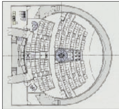
Farklı iki temel planetarium mimarisine ait örnek kesit ve planlar. Solda geleneksel yatay kubbe tipi, sağda, multimedya uygulamalarına daha açık, eğik kubbe tipi görünüyor. Her ikisinin de birbirine göre üstünlük ve zayıflıkları var.
