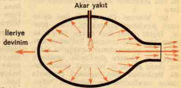
Şekil No. 3 b: Çıkan zerrecikler ileri devinimi oluştururlar
