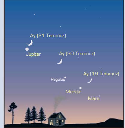
19-21 Temmuz akşamları batı ufku
