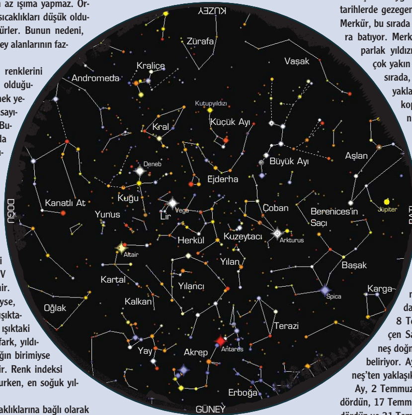
1 Temmuz saat 23:00; 15 Temmuz saat 22:00; 31 Temmuz 21:00'de gökyüzünün genel görünüşü
