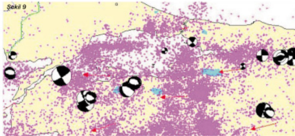
Şekil 8. Marmara denizi içindeki pull-apart basenlerinin en batıda yer alan Tekirdağ çukurluğunun dik normal fayları ve içinde yer alan genç çökeller gösterilmektedir (Wong vd., 1995) Şekil 9. Marmara Denizi ve çevresinin 1964-1994 yılları arasındaki deprem aktivitesi (ISC verileri). Kırmızı oklar GPS vektörlerini ve siyah beyaz toplar ise fay düzlemi çözümlerini göstermektedir (Straub ve Kahle, 1995).
