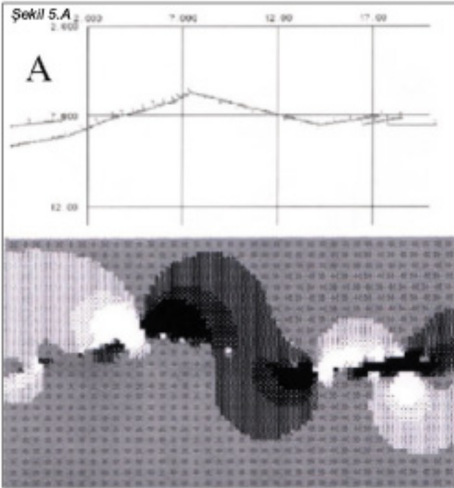
Şekil 5. Marmara Denizi'nde tek fay (A) veya kuzeyden ve güneyden sınırlayan iki fay (B) geçmesi durumunda elde edilen stres veya morfolojik dağılım. Her iki şekildeki dağılım bugünün Marmara Denizi içi veya dışı morfoloji ile uyuşmamaktadır.
