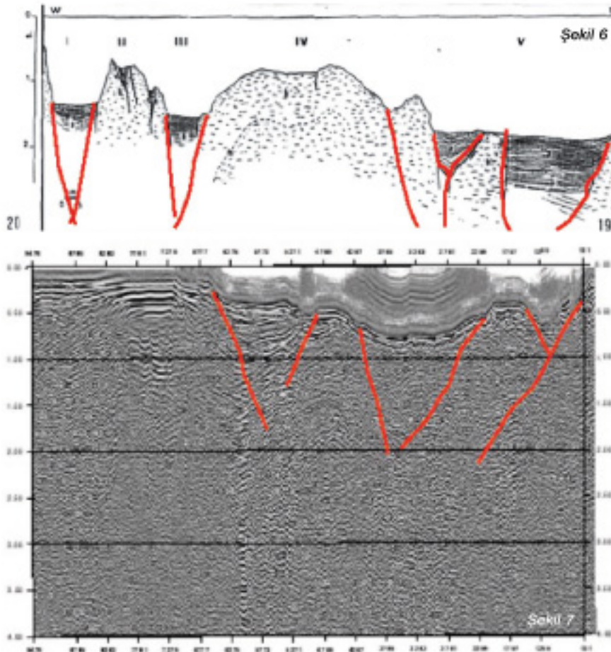
Şekil 6. Marmara Denizi içinde sıfır sismik yansıma profili basenleri sırtları arasında kalan transtansiyonel fayları göstermektedir (Ergün ve Özül, 1995'ten değiştirilerek alınmıştır). Şekil 7. Marmara Denizi orta sırta oblik K-G uzanımı sismik yansıma profili sırtın uzun eksenı boyunca genişleme olduğunu göstermektedir (Çetin vd. 1998'den değiştirilerek alınmıştır).
