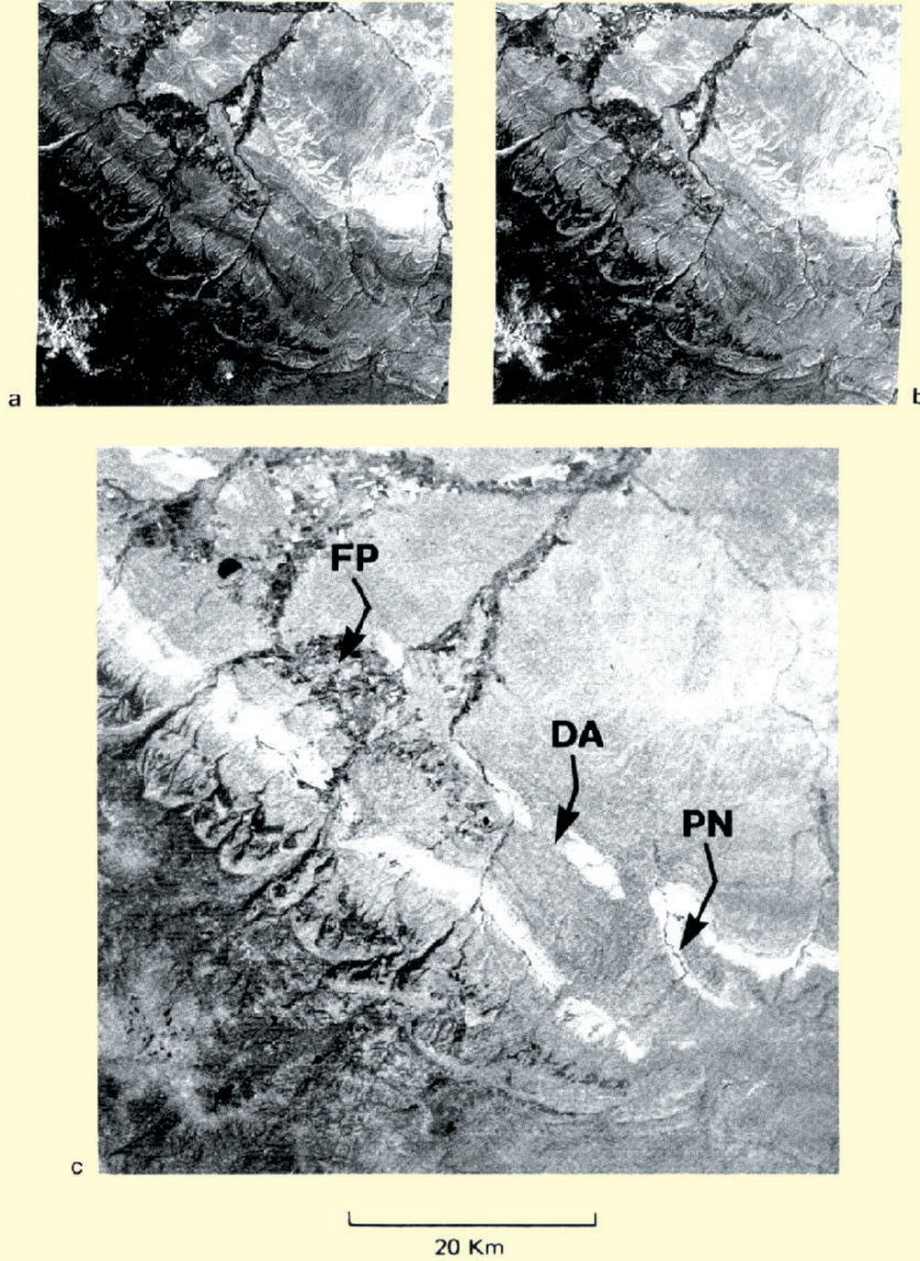
Şekil 5: (a ve b) Wind River Havzası'na ait bir görüntünün 4. ve 5. bantlarına ait görüntüler. (c) Bu iki bantın birbirine oranlanması (5/4) sonucunda ortaya çıkan görüntü. FP: Seldüzlüğü, DA: Dallas antiklinalı, PN: Dalımın ucu.
