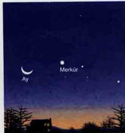
17 Aralık sabahı Ay ve Merkür
