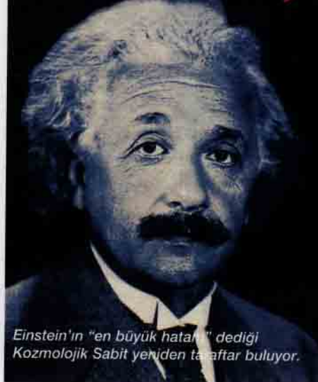
Formülünden şu sonuç çıkıyor: Evren genişliyor. Einstein bu "hatayı" düzeltmeye çalışmış, ta ki gökbilimciler bunu ispatlayana kadar.
