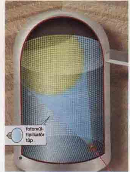
Yerin 1 km altındaki eski bir madende 50 000 ton arı su içeren silindirik bir sarnıçta içinde, herbiri 40 cm çapında, 13 000 fotomultiplikatör tüp, nötrino bir H veya O kuarkına çarpınca oluşacak Çerenkov ışımaları kaydetmeye hazırdır. Şekilde sağ alttan sarnıca giren bir nötrinin oluşturduğu mavi ışık konisi görünüyor.
