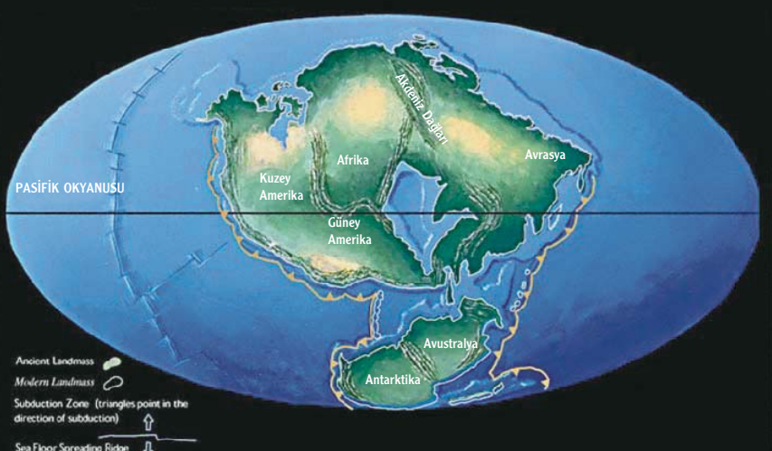
Atlantik Okyanusu küçüldükçe, kıtalar birleşerek yeniden bir süperkıta oluşturuyorlar: Pangea Ultima. Şekilde, Atlantik Okyanusu'nun kıtalar arasında sıkışarak oluşturduğu bir iç deniz de görülüyor.
