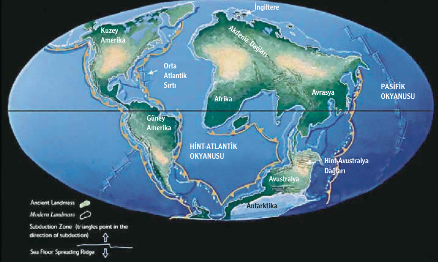
Güney ve Kuzey Amerika'nın doğu kıyıları boyunca ortaya çıkan dalma-batma bölgeleri, Atlantik sularının okyanus tabanıyla birlikte çekilmesi ve okyanusun küçülmeye başlayarak Amerika'nın, birleşmiş Avrupa-Afrika kıtasına yaklaşmasıyla sonuçlanıyor.
