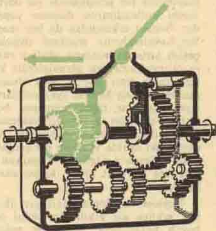
Şekil 3. Giriş ile çıkış milini doğrudan doğruya bağlayan 3. vites
