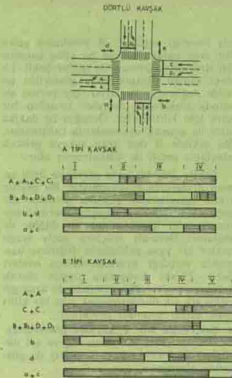
Şekil 4. Bir dörtlü kavşak (a) ve ilgili altı tip zaman diagramı
