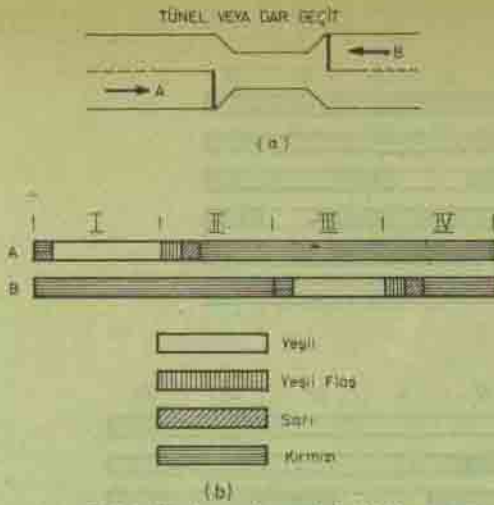
Şekil 1. Tünel veya dar geçit trafik idaretilmesi (a) ilgili zaman diagramı (b)
