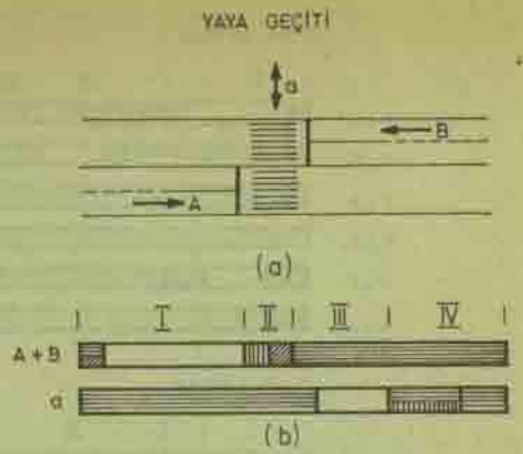
Şekil 2. Yaya Geçiti (a) ve ilgili zaman diagramı (b)
