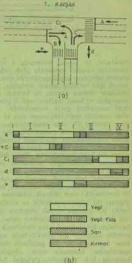
Şekil 3. Bir T kavşağı (a) ve ilgili zaman diagramı (b)
