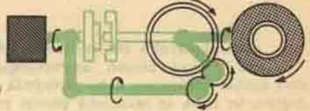
Şekil 2. 2. vitesde çalışan şanzuman
