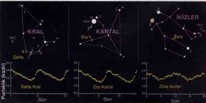
Yukarıda, üç sefid türü değişken yıldızın ışık eğrileri görülmüyor. Bu ışık eğrileri, John Isles tarafından çıplak gözle yapılan gözlemler sonucu elde edilmiştir.
