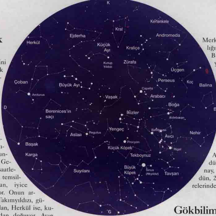
15 Mart 1998 Saat 21 00 'de gökyüzünün genel görünüşü
