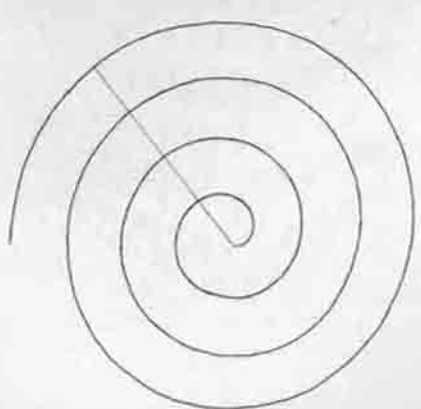
Arşimed spirali
