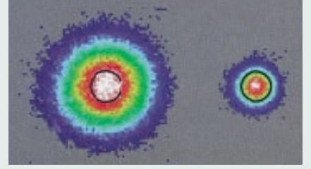
Süper soğutulmuş gazın sıcaklığı Fermi sınırından düşüğe (sağda), Fermi yüzeyinde (siyah halkalar) daha fazla atom birikiyor. Beyaz renk en yüksek atom yoğunluğunu, mavi-siyah ise en düşüğünü gösteriyor. Daha sıcak olan soldaki bulutta 2,5 milyon, neredeyse mutlak sıfırdaki sağ buluttaysa 0,78 milyon atom var. Bunda atomlar buharlaştırarak soğutma tekniği nedeniyle azalmış.
