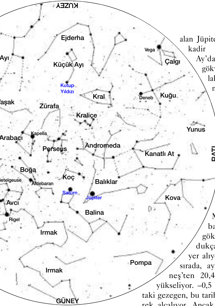
15 Aralık 1999 Saat 21 00 'de gökyüzünün genel görünüşü
