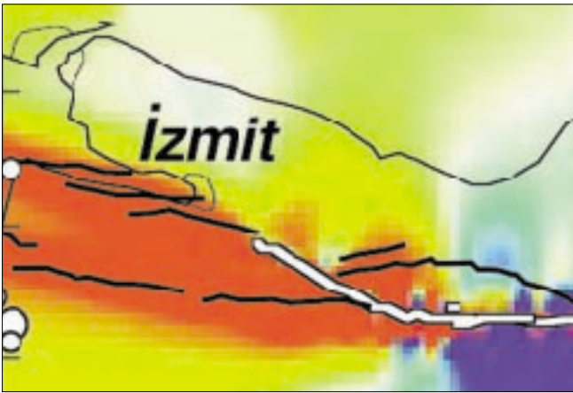
Şekil 4. Kuzey Anadolu fayı üzerinde 1939-1967 deprem göçü sırasında meydana gelen kırılma stresi dağılımı. Bu şekilde 17 Ağustos depremi öncesinde İzmit körfezinde kırılma stresi artışı görülürken Düzce fayında da azda olsa bir stres azalması hesaplanmıştır (mavi alan). Bu da 17 Ağustos depreminin Gölyaka'da kalması ile uyumludur (Stein, Barka ve Dietrich, 1997).
