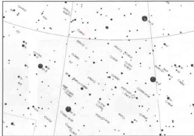
SKY ATLAS 2000.0 yıldız atlasından alınan bu bölüm, Büyük Ayı Takımyıldızı'nın (Büyük Kepçe) kepçesini gösteriyor. Atlasta, yıldızların hem Falmsteed numaraları, hem de Bayer harfleri; gökadalara ve Baykuş Bulutsusu'nun NGC numaraları, ayrıca bu gök cisimlerinden Messier Kataloğunda yer alanların Messier numaraları verilmiştir.
