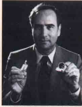
Fotonik devrimine yol açan ilk büyük gelişme Theodore Maiman'ın geliştirdiği lazereydi. İkinci önemli gelişmeye ise fiber optik teknolojinin doğuşu oldu.
