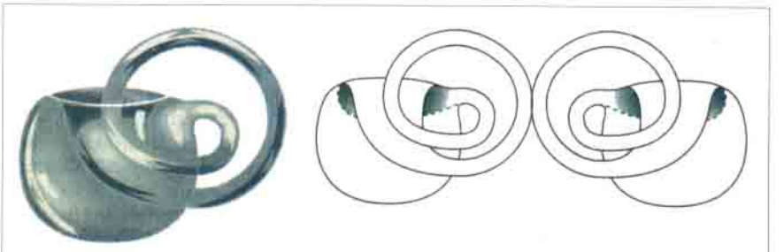
Ouslam kabı: Şişenin boynu iki spiral halka yapar, dikine ortadan kesilince her biri 3 burmalı iki Möbius bandı oluşur (noktalı çizgiler görmeyi kolaylaştırmak için eklenmiştir).
