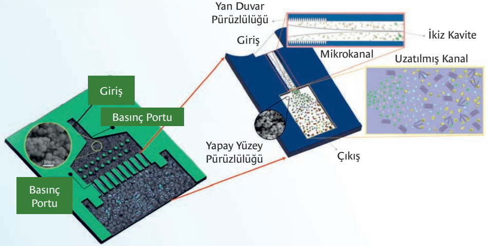
Mikrokirleticilerin sudan uzaklaştırılmasında kullanılan hidrodinamik kavitasyon reaktörlerin çalışma prensibi
