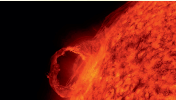
30 Mart 2010'da Solar Dynamics Observatory uydusu tarafından kaydedilen bu ardışık görsellerde bir Güneş patlamasının aşamaları görülüyor.
