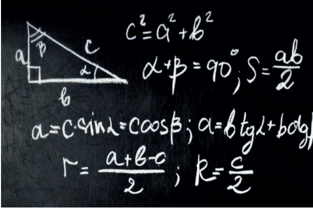
Pisagor teoreminin temsili gösterimi
