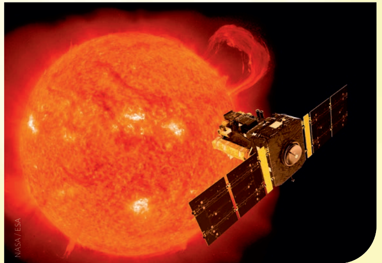
ESA ve NASA ortaklığıyla geliştirilen SOHO uydusu, 1996 yılından bu yana Güneş'i sürekli bir şekilde izleyerek iç yapısı ve atmosferiyle ilgili veri topluyor.
