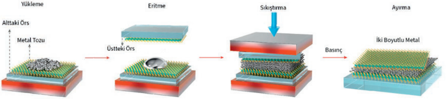
İki boyutlu metallerin üretim süreci
