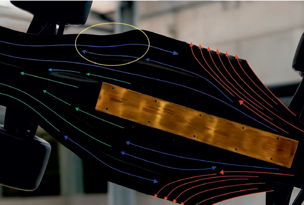
Aracın tabanında Venturi tünelleri olarak bilinen oyuklar hava akışını yönlendirir
