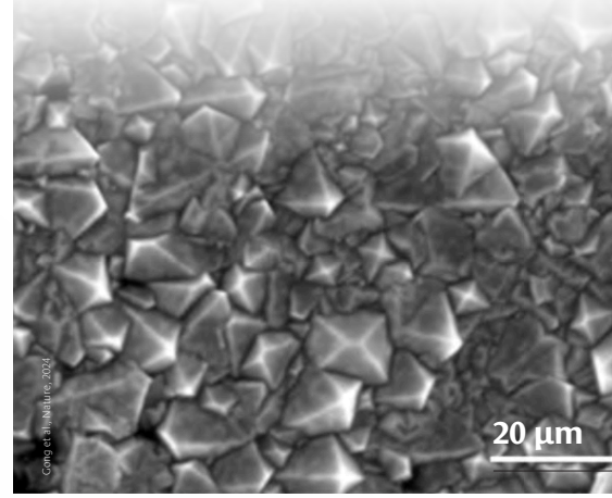
Sıvı metal içinde büyütülen ince elmas katmanının taramalı elektron mikroskobu görüntüsü
