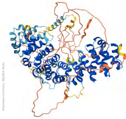
Bir proteinin AlphaFold3 kullanılarak oluşturulmuş üç boyutlu yapısı
