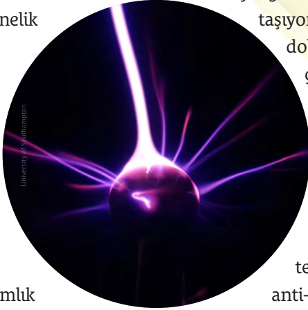
Kuantum kütleçekimi etkisindeki bir parçacığı gösteren temsili bir çizim
