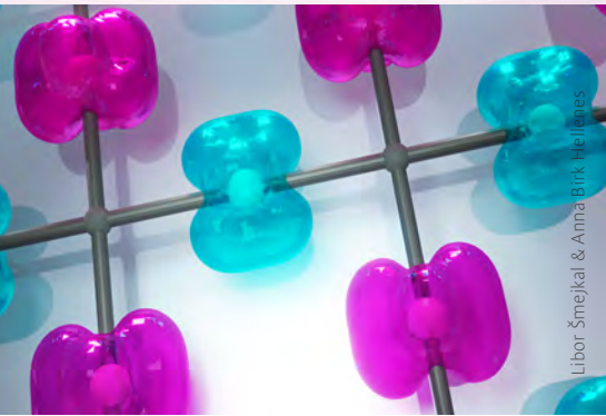
Bir altermanyetik malzemede, komşu elektronlar zıt yönlerde (farklı renklerle temsil edilen) dönüyor ancak farklı yönelimlere sahip (şekillerin farklı yönelimleriyle temsil edilen) atomik ölçekteki yapıların içinde bulunuyor.
