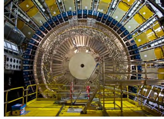
CERN'deki ATLAS detektöründen bir görüntü
