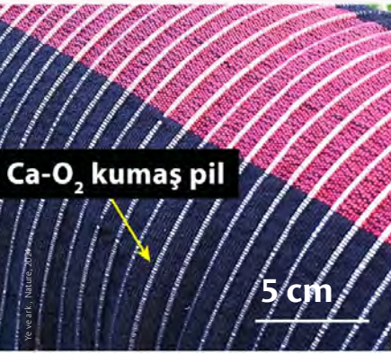
Solda \text{Ca-O}_2 yapılı pil liflerinden yapılan enerji depolayıcı kumaş, sağda bir cep telefonunu şarj etmekte olan bir kumaş pil
