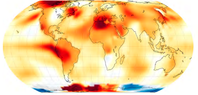
2023'ün temmuz ayındaki küresel sıcaklıkların mevsim normalleriyle (1951-1980 ortalaması) karşılaştırıldığı bir grafik. Kırmızı renk normalin üstünü, mavi renk normalin altını temsil ediyor.
