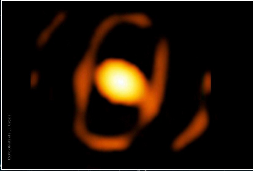
WOH 64 süper dev yıldızının dört büyük çaplı teleskopla elde edilmiş görüntüsü
