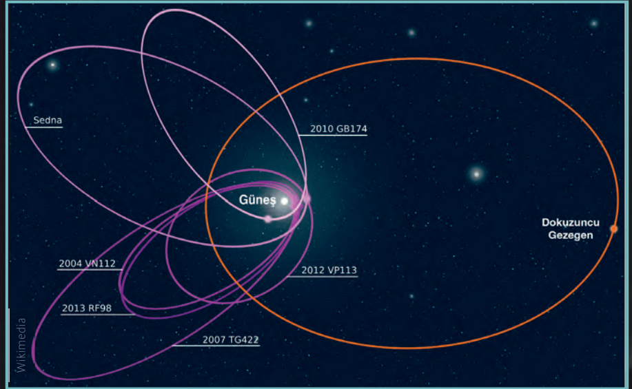
Güneş sisteminde, yörüngeleri Neptün'ün ötesinde bulunan, bilinen en uzak altı nesnenin yörüngeleri belirli bir yönde hizalanmış durumdadır. Ayrıca bu altı nesnenin yörüngelerinin eliptikliği benzerdir ve bilinen gezegenlerin yörüngelerinin bulunduğu tutulum düzlemine göre yaklaşık aynı açığı yapar.
