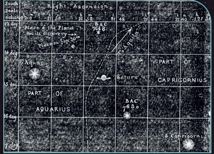
10 Ekim 1846'da The Illustrated London News adlı dergide yayımlanan bu görselde, daha sonra Neptün olarak adlandırılacak yeni bir gezegenin keşfi gösteriliyor. Yeni gezegenin keşfedildiği 23 Eylül'deki konumu ve 30 Eylül'de bulunduğu konum, görselin sol üstünde belirtilmiş.
