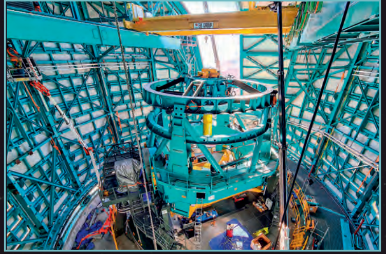
8,4 metre çapındaki aynaya ve geniş görüş açısına sahip Simonyi Tarama Teleskobu
