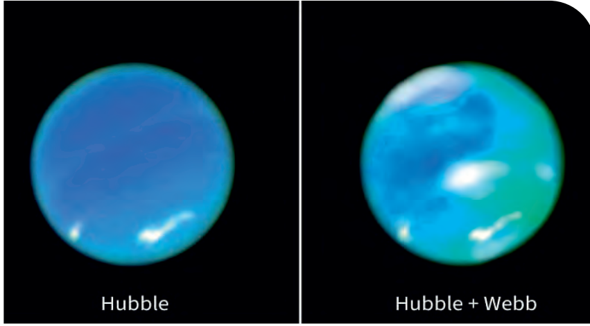
Neptün'deki auroranın görüntüsü. Sağdaki görsel Hubble ve James Webb verilerinin bir araya getirilmesiyle oluşturulmuş. Mavi gezegenin üzerindeki siyan renkli kısım auroranın meydana geldiği bölge.
