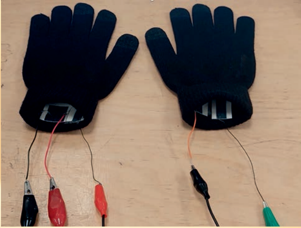
Algılama testi için e-tekstil örnekleri ve elektrik devre bağlantıları yapılmış olan eldivenler.
