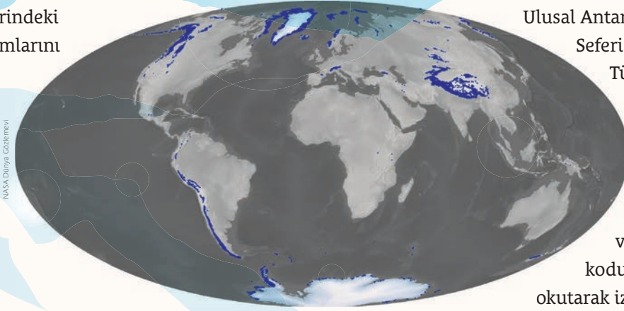
2013'te ilk kez oluşturulan Dünya Buzul Haritası'nda buzullar koyu mavi, buz örtüleri açık mavi-beyaz, okyanuslar gri, kıtalar ise açık gri ile renklendirilmiştir.
