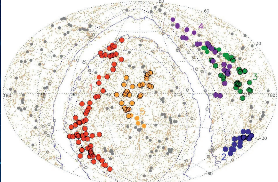
Bu şema yeni keşfedilen süper yapıları gösteriyor. Quipu (kırmızı) yerel evrende keşfedilmiş en büyük yapı. Diğerleri de Shapley (mavi), Serpens-Corona Borealis (yeşil), Hercules (mor) ve Sculptor-Pegasus (sarı).
