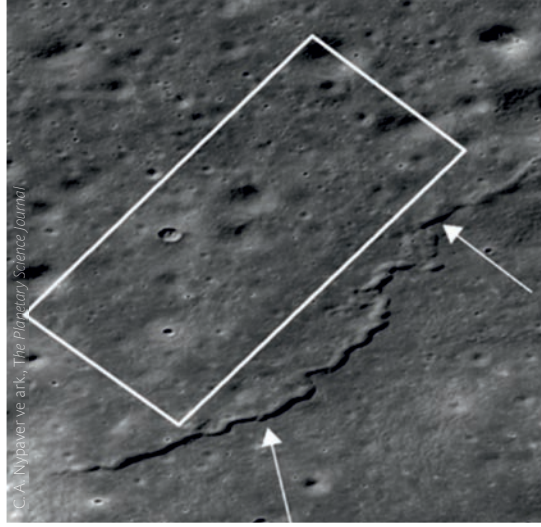
Ay'ın Dünya'ya uzak yüzündeki çıkıntılar ve bu çıkıntılarının yaşını tahmin etmek için kullanılan krater sayma bölgesi
