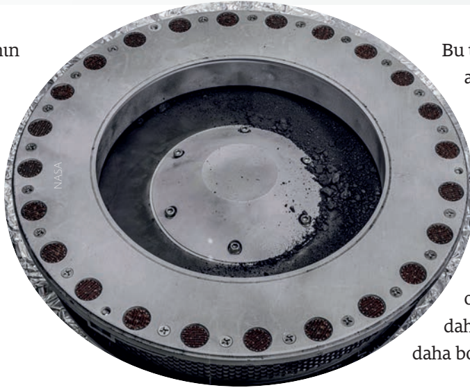
OSIRIS-REx uzay aracının örnek toplama bölümünün dış kısmı. Fotoğrafın orta bölümün sağında Benu Asteroiti'nden alınan örneklerin bir kısmı görünüyor.
