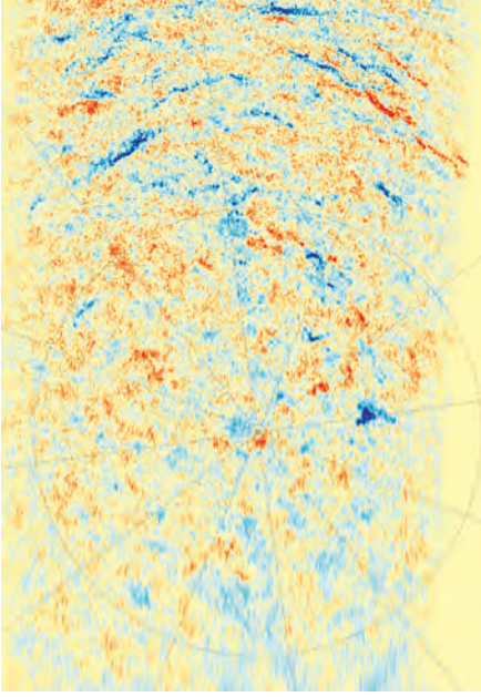
Güneş'in güney kutbundaki manyetik alanın haritası. Görselde manyetik kuzey kutupları kırmızı, manyetik güney kutupları ise mavi renkle işaretlenmiş. Daha koyu tonlar daha güçlü bir manyetik alanın varlığını gösteriyor.
