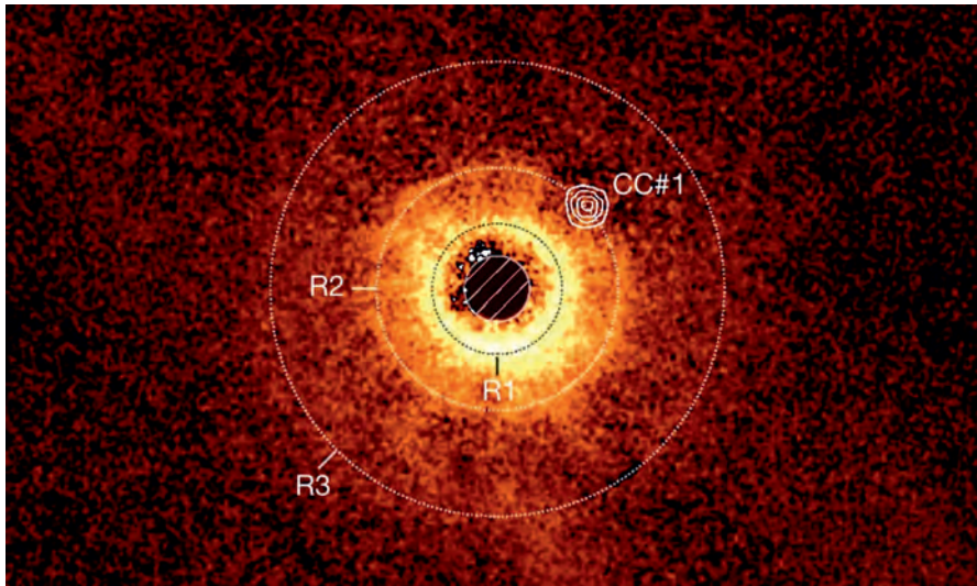
James Webb Uzay Teleskobu'nun kızılötesi kameralarını TWA 7 yıldızına doğrultarak elde ettiği görüntü. Yoğun madde bulutuyla çevreli olan yıldızın ışığı, koronagraf cihazı tarafından maskeleniyor. Keşfedilen ötegezegen, R2 halkası civarındaki boş bölgenin içinde (CC#1) yer alıyor.
