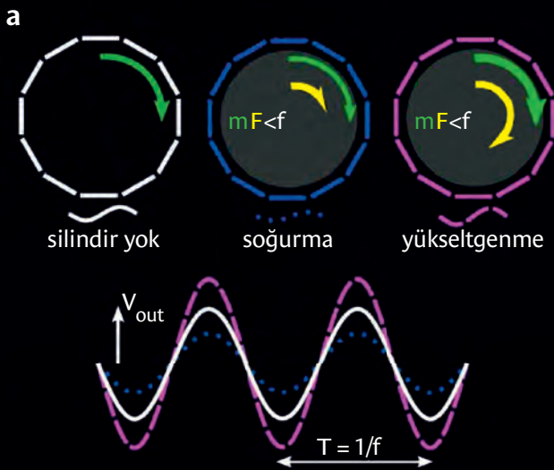
Süperışınmanın ortaya çıkması için gerekli koşullar (a) ve kara delik bombası düzeneğinin şeması (b).
