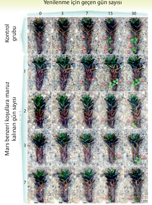
Görsele uygun koşullar altına alınan yosunların 30 gün içerisinde büyümesindeki değişimi yeni dal ve yapraklar oluşumlarıyla fark etmek mümkün. Kırmızı oklar, yeni filiz oluşumlarını işaret ediyor. Kontrol grubu ise Syntrichia caninervis yosununun uygun koşullarda 30 gün boyunca büyürken geçirdiği değişimi gösteriyor.
