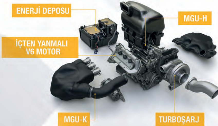
Modern MGU-K jeneratör motor ünitesi
