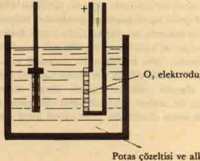
Şekil No. 5. JUSTI - WINSEL sıvı yakıt hücresi
