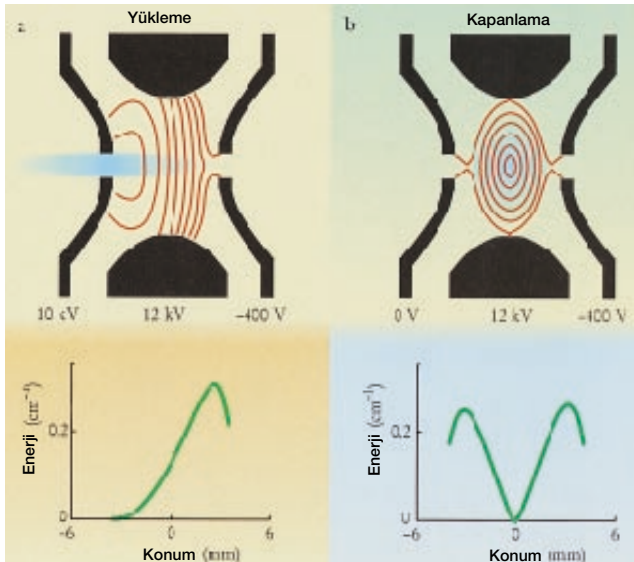
Şekil 2 Elektrik alanından kapalı. a) Kapana giren dipolar moleküller (mavi bulut) keskin bir şekilde değişen bir elektrik alanının (kırmızı çizgiler) etkisi altında kalırlar. Elektrik alanına ters yönde dipol momenti olan moleküller yavaşlar. Altta grafik potansiyel enerjiyi konumun fonksiyonu olarak vermektedir. b) Moleküller kapanın içine girince alan konfigürasyonu (üstte) molekülleri kısıran bir potansiyel kuyusu (altta) oluşur.
