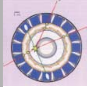
ATHENA ekibinin deneyinde ortaya çıkan antihidrojenin dolaylı kanıtı: Penning tuzacı içinde oluşan, antihidrojen tuzak çeperinde maddeyle etkileşerek yok oluyor (sarı yıldız). Antiprotonun, protonla etkileşmesi sonucu 3 adet pion ortaya çıkıyor ve dedektörün iç kesimindeki silikon bantların iç ve dışı belirleniyor (yeşil daireler). Bu daireleri birleştiren doğrular, çarpışmanın olduğu yeri gösteriyor. Antiproton çevresinde dolanan pozitronun, bir elektronla etkileşmesi sonucu oluşan gama ışın fotonlarıyla, dış dedektördeki sezyum iyodür kristallerinde saçılarak ışıma yapıyor (yeşil çizgiler).
