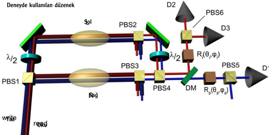
Deneyde kullanılan düzenek
