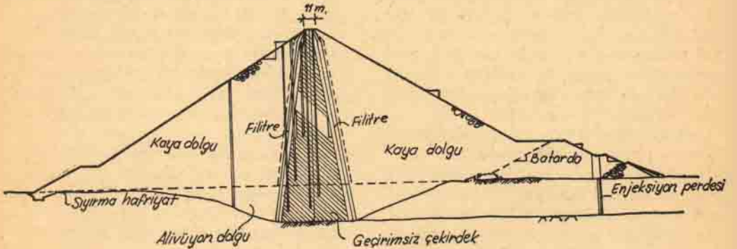
GÖVDE EN KESİT
