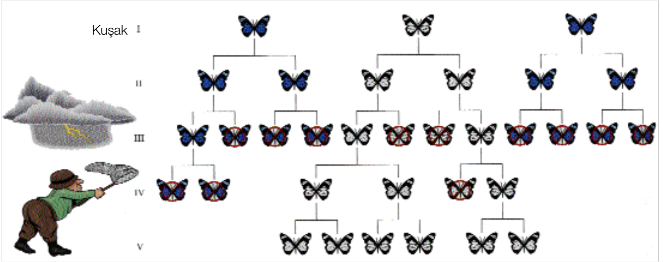
Küçük bir kelebek popülasyonunda rastlanabilecek genetik sürüklenmeye ilişkin kuramsal bir örnek. Her sembol mavi kanatlı (A alleli) ya da beyaz kanatlı (a alleli) döl vermek üzere çiftleşen iki kelebeği simgeliyor. İlk kuşakta 6 kelebekten 4'ü mavi kanatlı. İkinci kuşakta gen frekanslarında hiçbir değişiklik yaşanmaz. Üçüncü kuşakta meydana gelen bir fırtına ikisi hariç mavi kanatlıların hepsini, beyaz kanatlılarınsa yarısını öldürür. Sağ kalanlar tekrar ürer, ancak gen frekansları artık değişmiştir. Bir kelebek koleksiyoncusu mavi kanatlılardan (A alleli) geriye kalan dört taneyi ve beyaz kanatlılardan iki taneyi koleksiyonuna katar. Rastlantısal bazı nedenlerden ötürü başta az olan a alleli, dördüncü kuşakta hakim gen haline gelmiş, A alleliyse popülasyondan silinmiştir.
