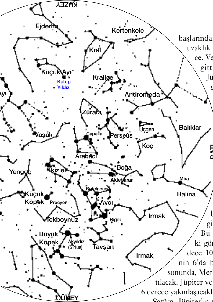
15 Şubat 1999 Saat 21 00 'de gökyüzünün genel görünüşü
