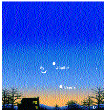
18 Şubat akşamı Ay ve Jüpiter ve Venüs
