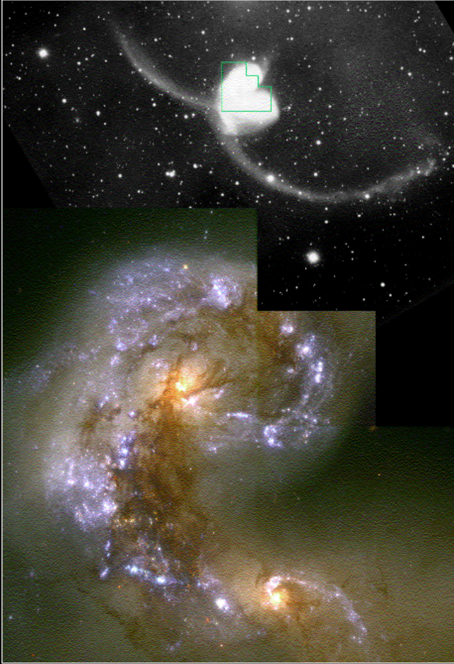
Çarpışan gökadalar: Anten Gökadaları (NGC 4038 ve NGC 4039) olarak bilinen bu gökadalar, biçimlerinden dolayı bu adı almışlar. Yaklaşık 63 milyon ışık yıl uzaklıkta yer alan bu iki gökada bir-biriyle çarpışıyor. Hubble, bu fotoğrafı 20 Ocak 1996'da çekti.
