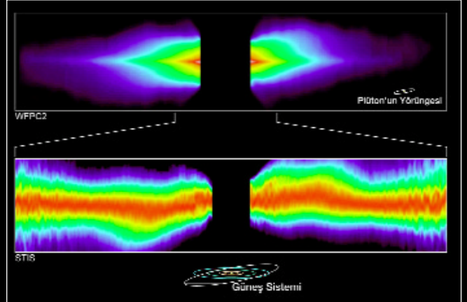
Beta Pictoris: Bu yıldız, gezegenlere sahip olabilecek yıldızlara gösterilebilecek en iyi örneklerden biridir. Yandaki görüntülerde, Beta Pictoris sistemindeki gaz ve toz diski kenardan görülüyor. Kırmızıdan mora değişen renkler, azalan parlaklığı gösteriyor.
