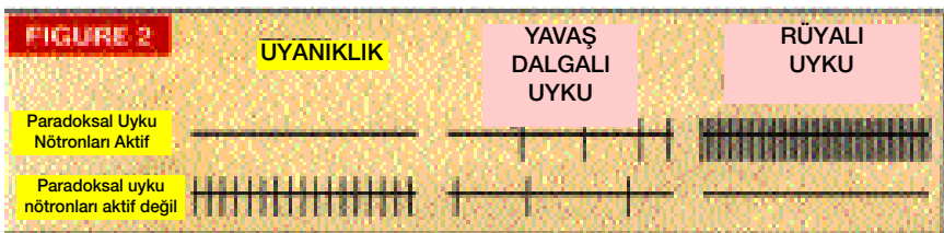
Rüyalı uyku sırasında bazı nöronlar (SP-ON) etkinleşir, diğer nöronlar (SP-OFF) ketlenir. Uyanıklık sırasında bunun tersi olur.
