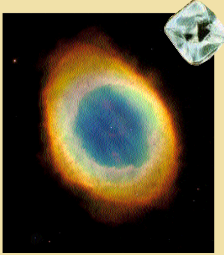
Çalgı takımıyıldızındaki Halka Bulutsusu'nun Hubble teleskopu tarafından çekilmiş görüntüsü.
