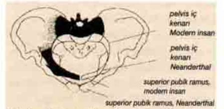
Modern insan ve Neanderthal pelvis farkları
