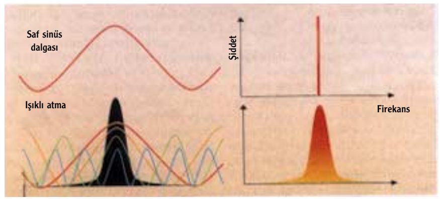
İşıklı bir atma, "saf" sinüs biçiminde bir dalganın tersine, içinde pek çok frekansı barındırır. Atmanın tepe değeri, bu atmayı oluşturan bütün frekansların birbiriyle aynı fazda oldukları noktadır. Atma ne kadar ince ve yerelse, tayfı da o denli geniş demektir. Atmanın yer değiştirme hızı, sinüs biçimli dalgaların hızına, ancak eşzamanlı (senkronize) olarak yer değiştirdiklerinde, yani kırma indisi frekansla değişmediğinde eşit olur.
