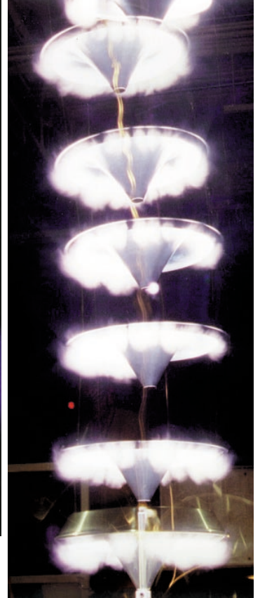
Minyatür bir hafif uzay aracı, 10 kilowattlık bir lazer enerjisiyle 30 m yükseğe çıkarılabiliyor. Daha büyük tasarımlar, araca yörüngeye oturabilecek kadar büyük bir hız sağlayabilecek.
