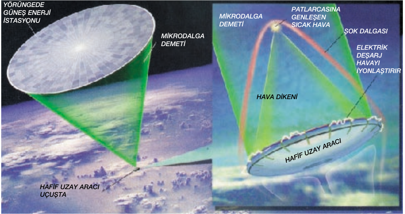
Yörüngedeki bir güneş enerji istasyonu (üst sol), manyetohidrodinamik itkiyle çalışan hafif bir uzay aracına (sağ) mikrodalgalar şeklinde enerji yollayabilir. Uzay aracı mikrodalga enerjisini odaklayarak bir "hava dikenini" yaratır; bu diken sürtünme direncini azaltır. Hafif uzay aracının kenarındaki elektrodlar havayı iyonize ederek itkiye katkıda bulunur.
