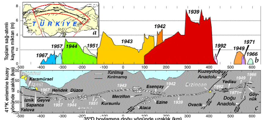
a) Kuzey Anadolu Fayı kalın olmak üzere, Türkiye'deki diri faylar. b) Büyüklüğü 6.7 ve üzerinde olan depremlerden kaynaklanan sağ-atımlı kaymaların toplam uzunluklarının grafiği. c) Kuzey Anadolu Fayı üzerindeki depremler ve bunların kırdığı fay kısımları.
