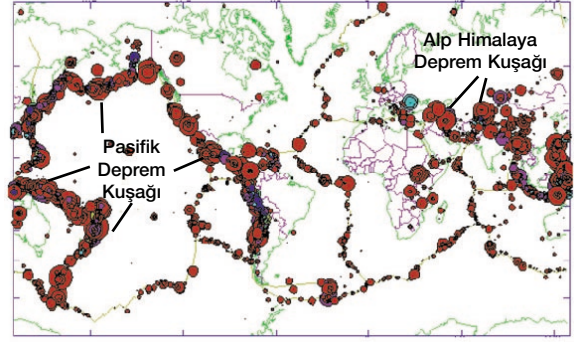
Yerkabuğunu oluşturan levhaların sınırları, depremlerin yoğunlaştığı bölgelerdir. Özellikle levhaların birbirine yaklaştığı sınırlar, daha çok büyük depremlerin sıkça gözlemlendiği, iki büyük deprem kuşağıdır. Bunlardan büyük olanı Pasifik Deprem Kuşağı, diğeri Alp-Himalaya Deprem Kuşağı adını alır.
