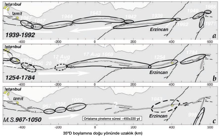
Kuzey Anadolu Fayı üzerinde gerilme aktarımının "tarih öncesi". 1939'dan öncesine ait, tarihsel kayıt incelemesiyle derlenmiş deprem sıralamaları. İşaretlenmiş alanların kesinlik taşımadığı unutulmamalı.
