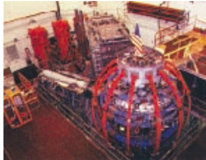
Ateş topu: Princeton'daki Ulusal Küresel Torus Deneyi.
