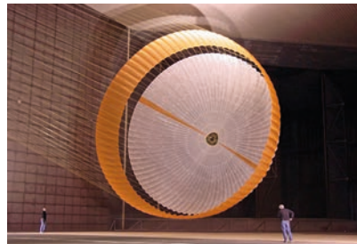
Kapsülün Mars yüzeyine inişi sırasında erişilecek yüksek hızın frenlenmesinde kullanılacak paraşüt
