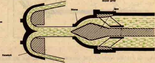
Şekil No. 4 PELTON türbini ayar mekanizması (çift kademeli ayar pektli)
