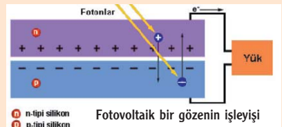
Fotovoltaik bir gözede elektrik alanının etkisi
