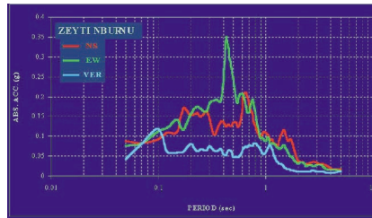
Şekil 2. 17 Ağustos Kocaeli depreminde Zeytinburnu deprem istasyonunda güney-kuzey ve doğu batı doğrultusunda kaydedilen ivme kayıtları (solda). Şekil 3. Aynı depremde Zeytinburnu deprem istasyonunda kaydedilen ivme kayıtlarından hesaplanmış ve zemin hakim periyodu ile spektral büyütme gösteren mutlak ivme spektrumları (üstte).
