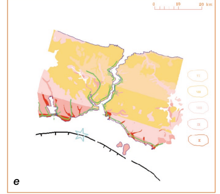
a) Senaryo depreminin bölgede sert zeminlerde yaratması beklenen deprem şiddeti. b) İstanbul otoyol şebekesi ana hatları senaryo depremi şiddet dağılımı haritası üzerinde gösterilmiştir. c) İstanbul doğalgaz şebekesi ana hatları senaryo depremi şiddet dağılımı haritası üzerinde gösterilmiştir. d) İstanbul'da şehir suyu şebekesinin ana hatları senaryo depremi şiddet dağılımı haritası üzerinde gösterilmiştir. e) İstanbul'da atık su şebekesinin ana hatları senaryo depremi şiddet dağılımı haritası üzerinde gösterilmiştir.
