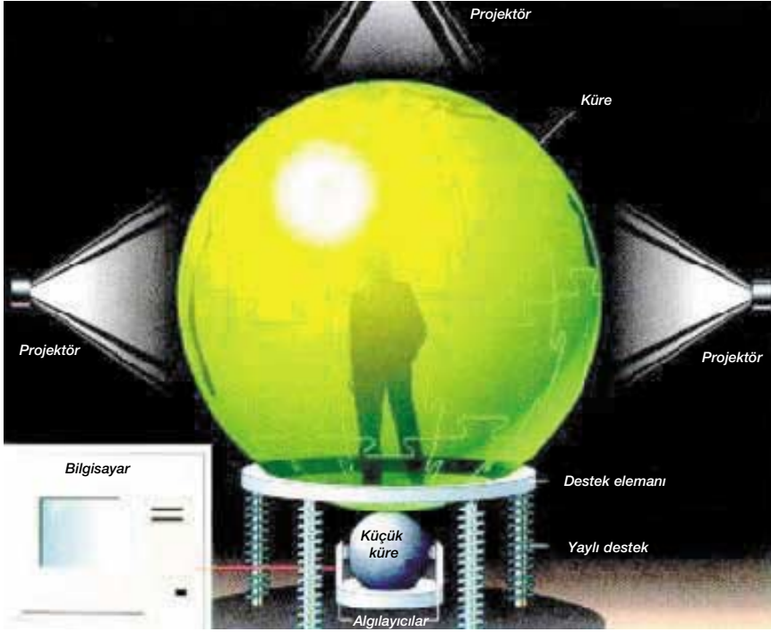
Sanal gerçeklik küresiyle hava yastıklı desteklerinin çalışma sistemi
