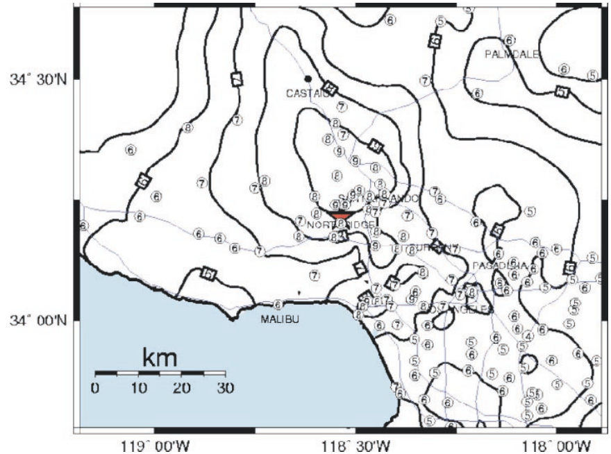
Kaliforniya'da 1994 yılında meydana gelen Northridge depremi için aletsel olarak üretilen eşşiddet haritasıyla, depremden sonra arazi gözlemlerinden elde edilen şiddet değerlerinin (dairele içindeki rakamlar) bir karşılaştırması gösteriliyor. Şekilde, aletsel ve gözlemsel şiddet değerleri arasındaki uyum, büyük bir depremin bir dakika sonra real-time deprem sistemleri tarafından sağlanacak bir aletsel şiddet haritasının yetkililer için ne kadar önemli olduğunu gözler önüne seriyor.
