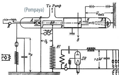
Wideröe'nün Ising'in kuramını kullanarak yaptığı ilk doğrusal hızlandırıcının doktora tezinde ver alan çizimi
