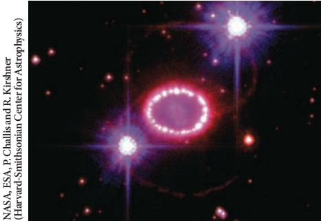
SN1987A'nın patlamasının 20. yıldönümünde Hubble Uzay Teleskobu tarafından gözlenmesi. Etrafındaki bulutsu genişlemeye devam ediyor. Astrofizikçiler hâlâ bulutsunun içinde oluşan hareketleri modellemek için uğraşıyor.
