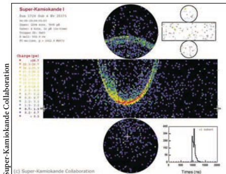
Super-Kamiokande'nin gözlemlediği bir müon-nötrinonun dedektörün içinde neden olduğu şok dalgasının (Çerenkov ışıması) fotoğrafı.
