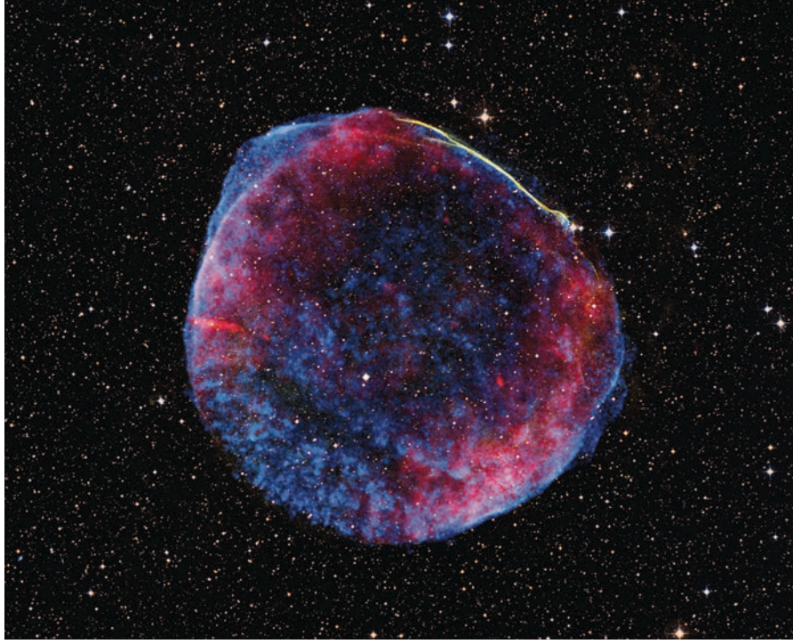
SN 1006 süpernovasının patlaması Dünya'dan MS 1006'da, Nisan sonunda gözlemlenmiş olsa da, bundan yaklaşık 7200 yıl önce gerçekleşmiş.
