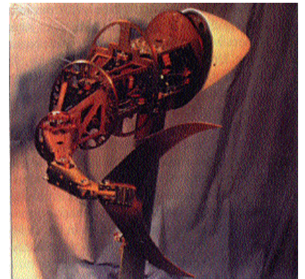
Istakoz robot (sol üstte) hem yürüyebiliyor hem de dönebiliyor. Tonbalığı robotunun (üstte) "kasları" onun gerçek bir balıkmış gibi dönmesini sağlıyor. Robot Hexapod (sol altta) engeli bir arazide bile rahatlıkla ilerleyebiliyor.
